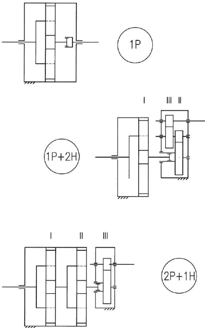
Fig.2. Schemele cinematice ale multiplicatoarelor instalațiilor energetice eoliene moderne
